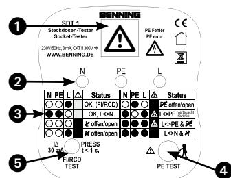
Joonis 1. Seadme esikülg
